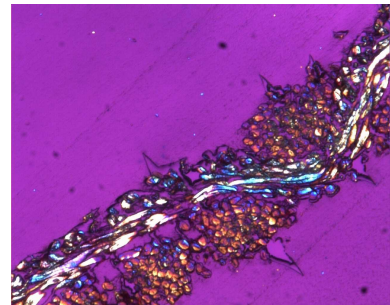
Ungenügende Infiltration
