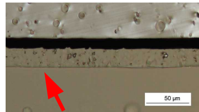
Guter Randschluss
